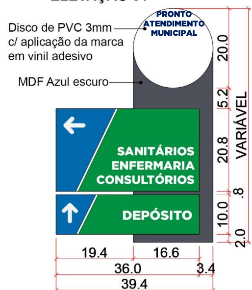
ELEVAÇÃO 02
