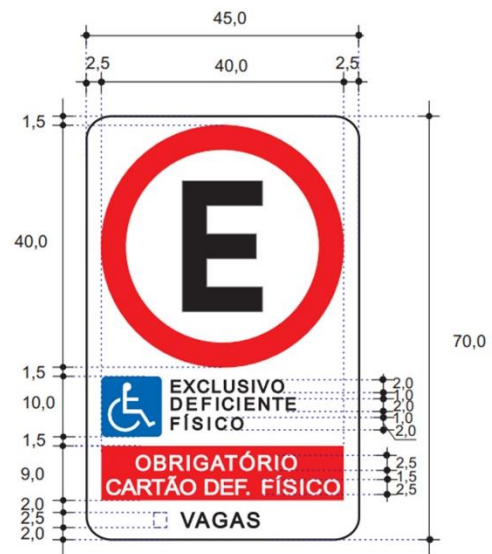
LAYOUT ESTACIONAMENTO DEF. FISICO
