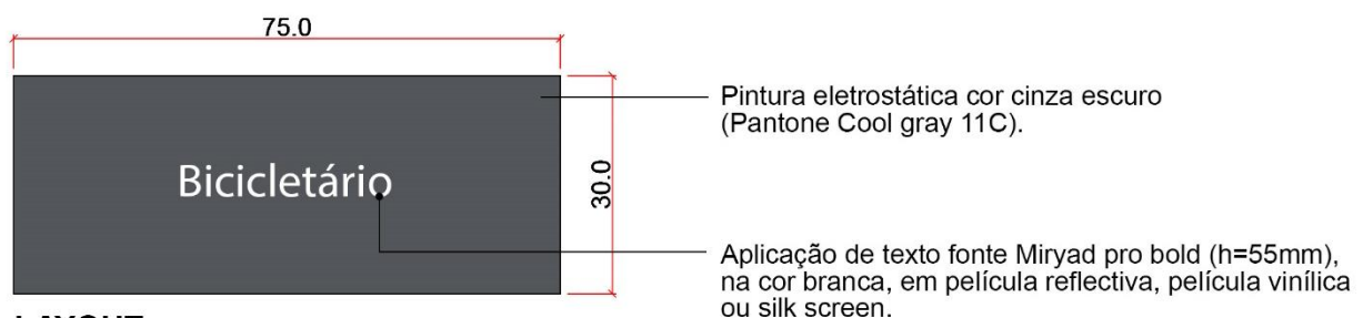
LAYOUT PLACA
